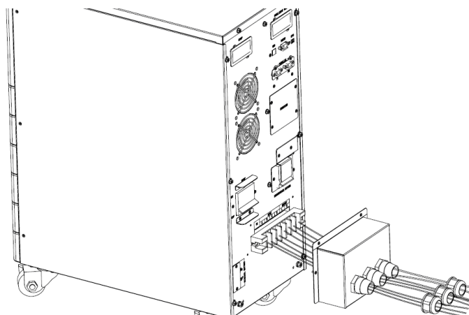
Подключение кабелей для ИБП 3110L
