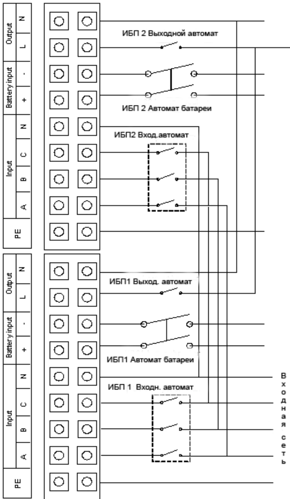
Схема соединений для 3115L, 3120L
