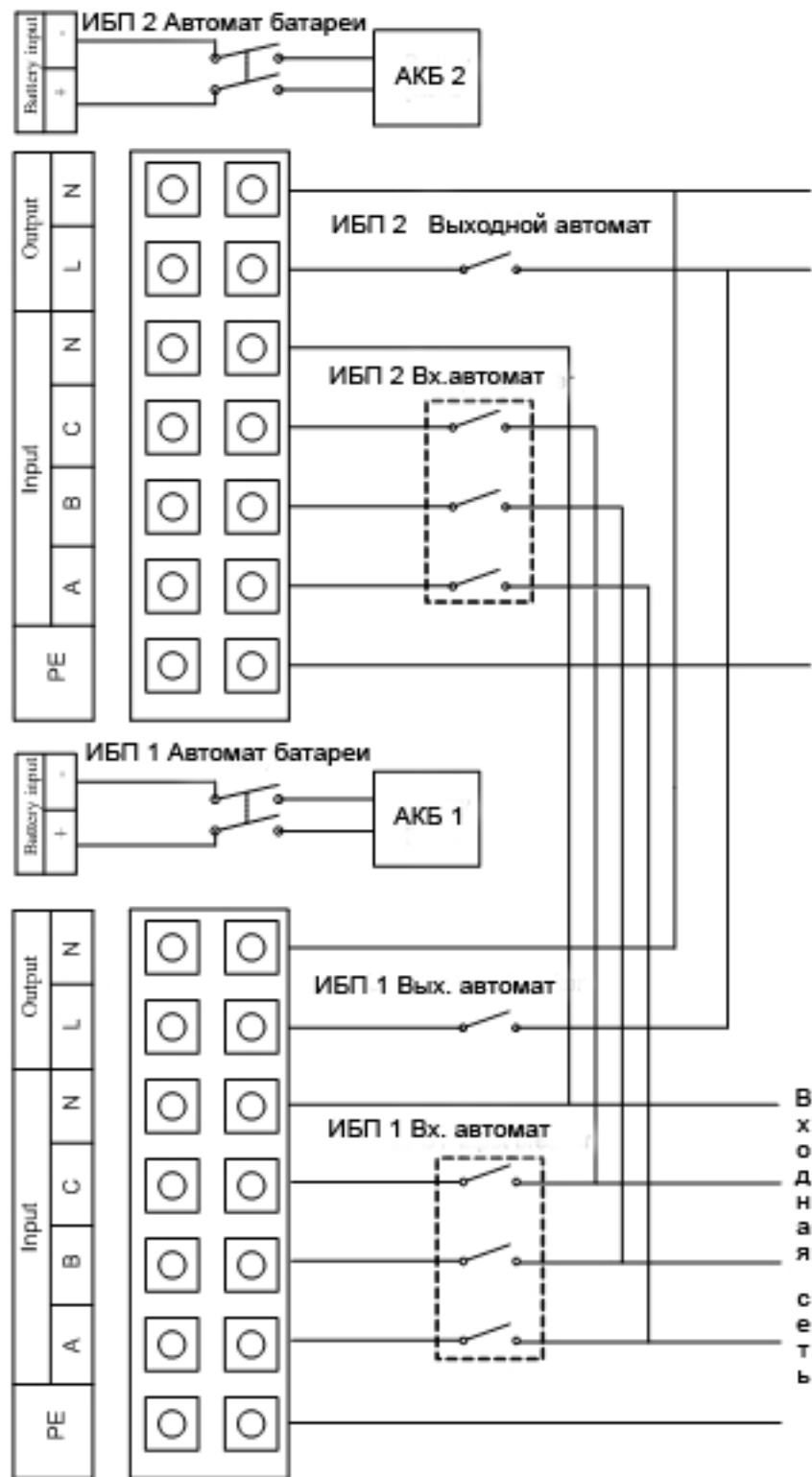
Схема соединений для 3110L
