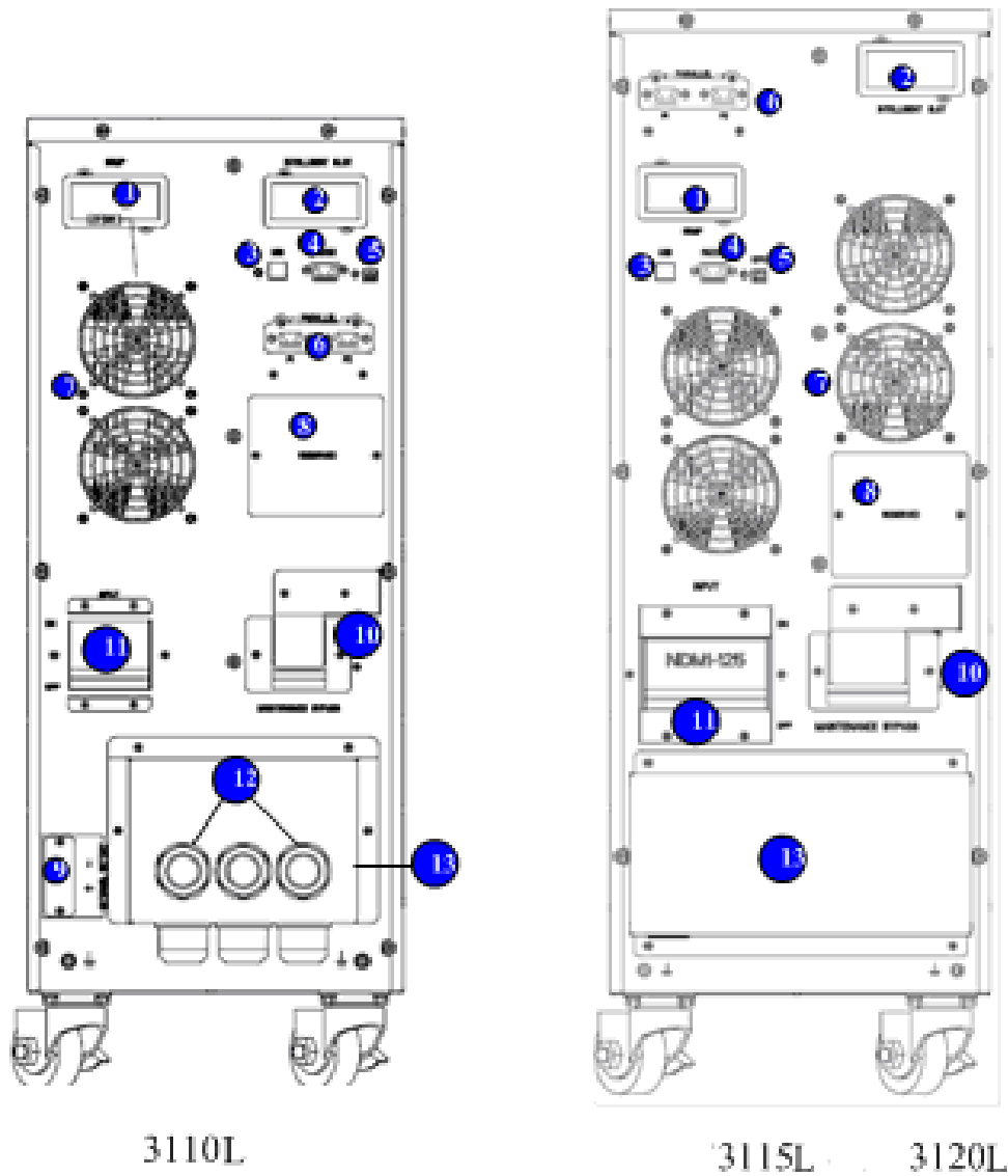
Задняя панель ИБП
